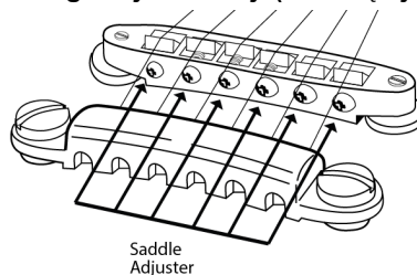
Źródło regulacji intonacji (dla każdej struny)
