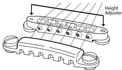
Vis de réglage de la hauteur
