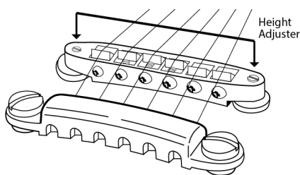
Höheneinstellschraube
