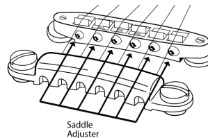
Intonatie instelschroef (voor elke snaar)
