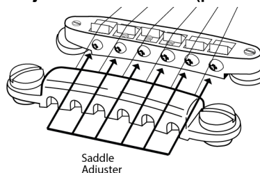
Tornillo de ajuste de entonación (para cada cuerda)
