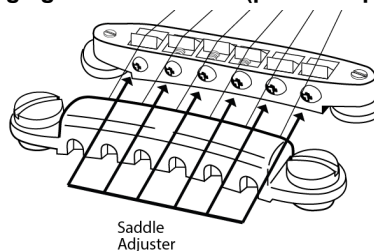
Vis de réglage de l'intonation (pour chaque corde)
