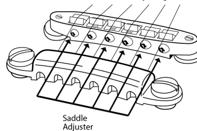
Intonationseinstellschraube (für jede Saite)
